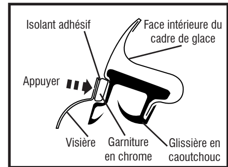
Coupe transversale de la visière en place
